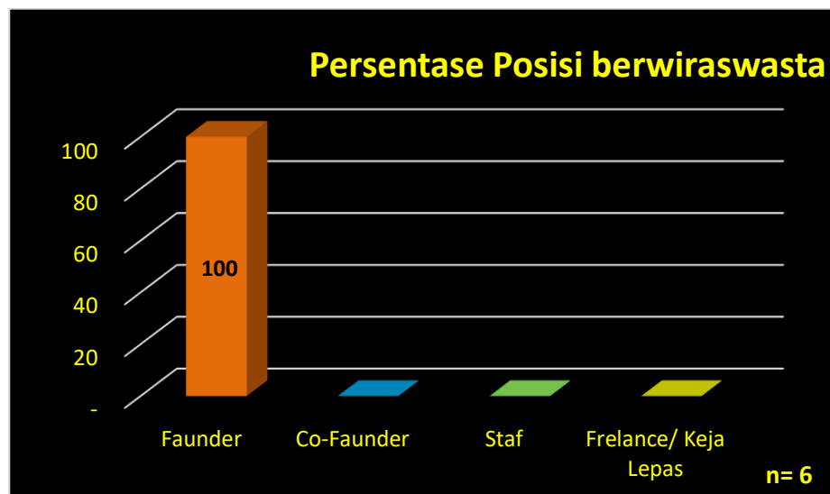
Gambar3. Posisi Bekerja
